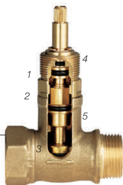
REGISTRO DE PRESSÃO DOCOL BASE 25140500 1/2" 25140600 3/4"
